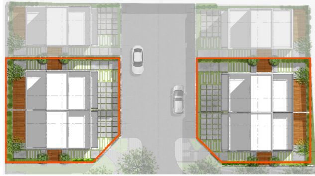
MẶT BẰNG TỔNG THỂ THE VILLAS THE VILLAS MASTER PLAN
